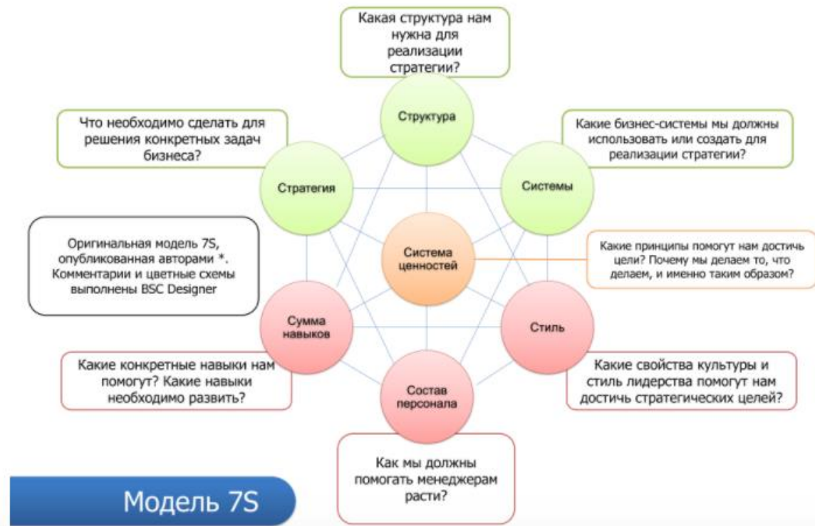
Рис. 3.14. – Модель 7-S
